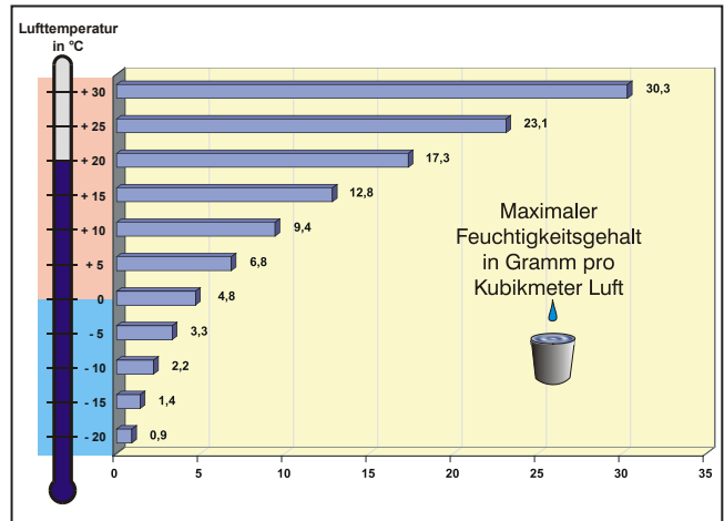
Maximaler Wasserdampfgehalt (= 100% relative Luftfeuchte) in Gramm pro \text{m}^3 Luft bei verschiedenen Temperaturen.
